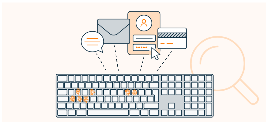
Figura 1.3: Keylogger
